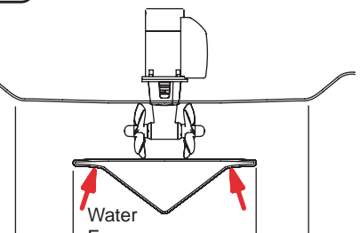
トンネル長を長く取って高速航行時の水圧からプロペラを保護する
