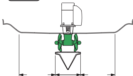
ギヤレグとプロペラはトンネルからはみ出さないこと
