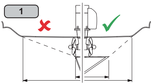
トンネル上部の長さ下部の長さの差が極端にならないようにすること。
