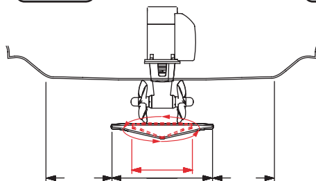
トンネル長を長く取ってプロペラとハルの間で循環する海水の吸い込みを防止する
